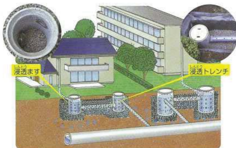
雨水浸透ますと浸透トレンチ
