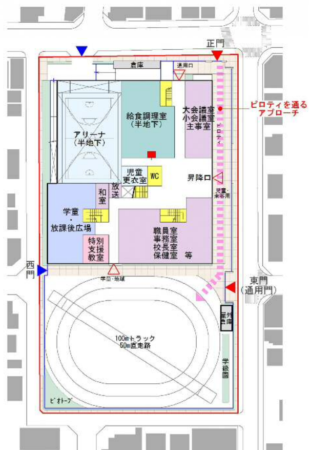
配置図兼1階平面イメージ
