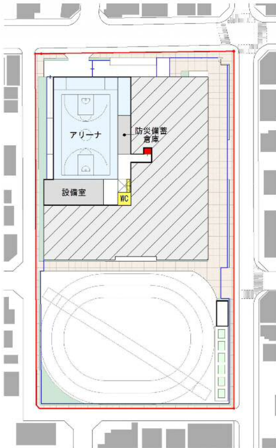
地下1階平面イメージ
