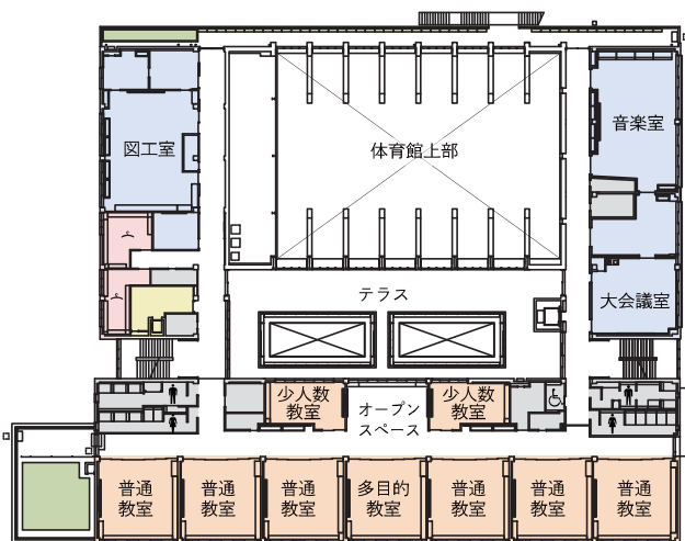
3階平面図
