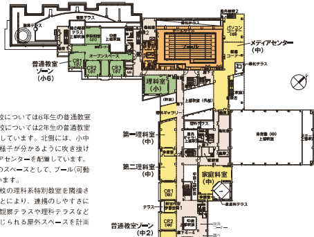
4階平面図
