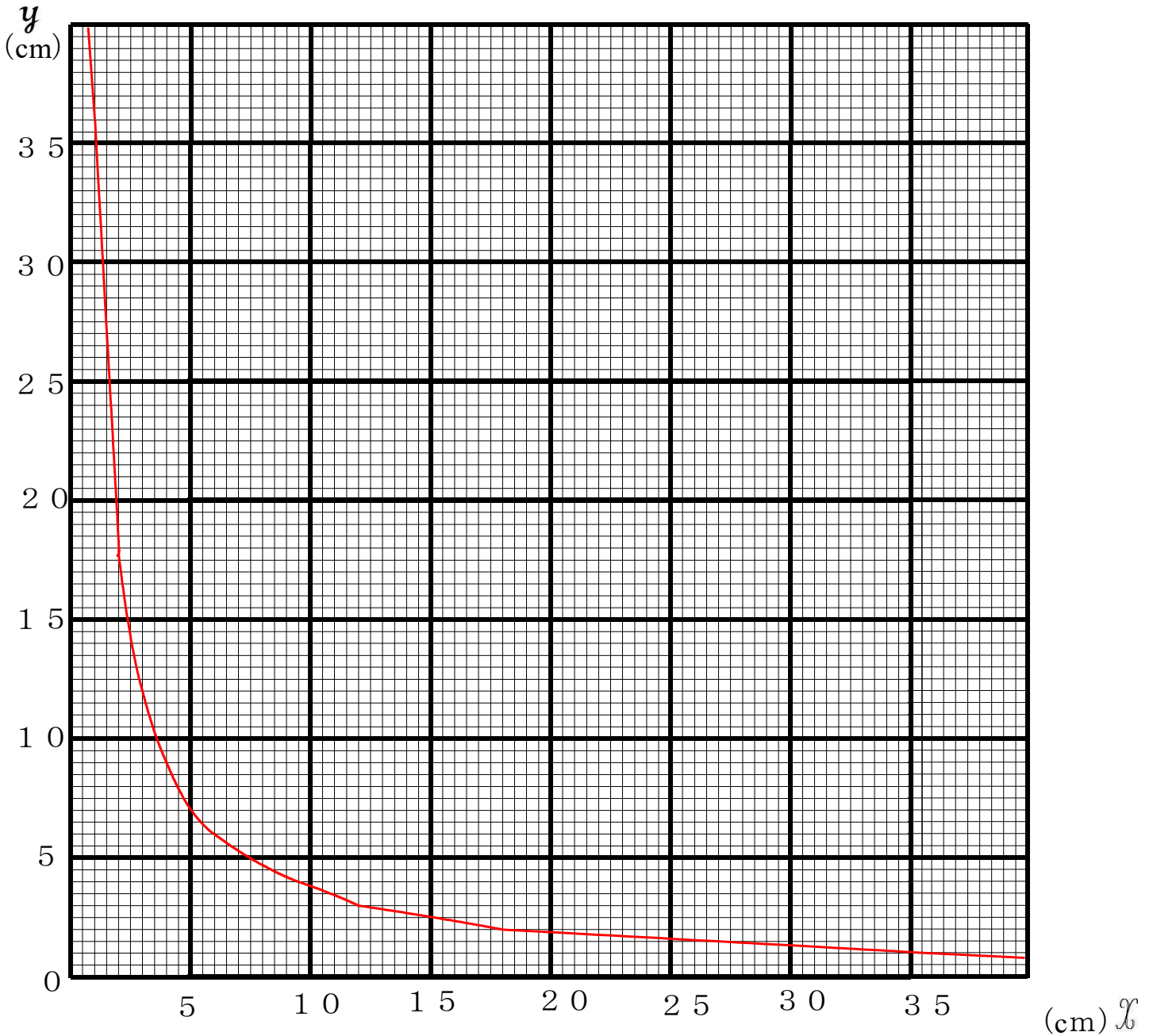
面積が 36 \text{ cm}^2 の長方形の縦の長さ x と横の長さ y
