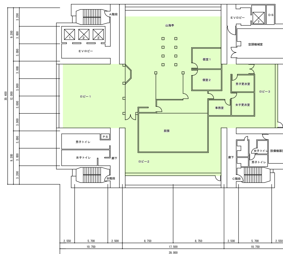
17階平面図
