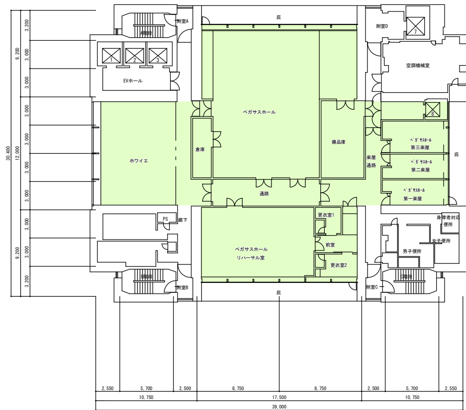
15階平面図
