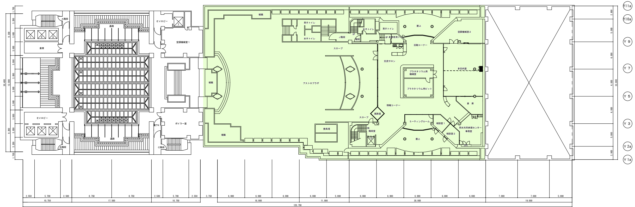
5階平面図
