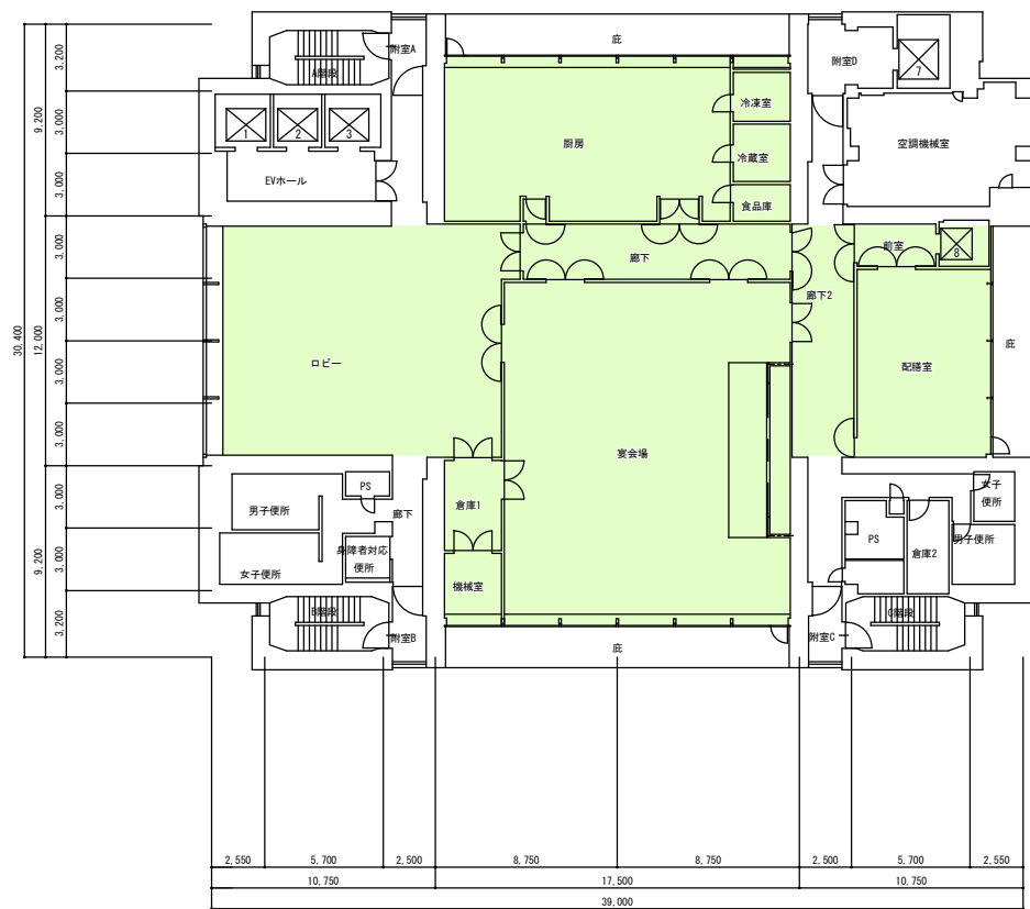
16階平面図
