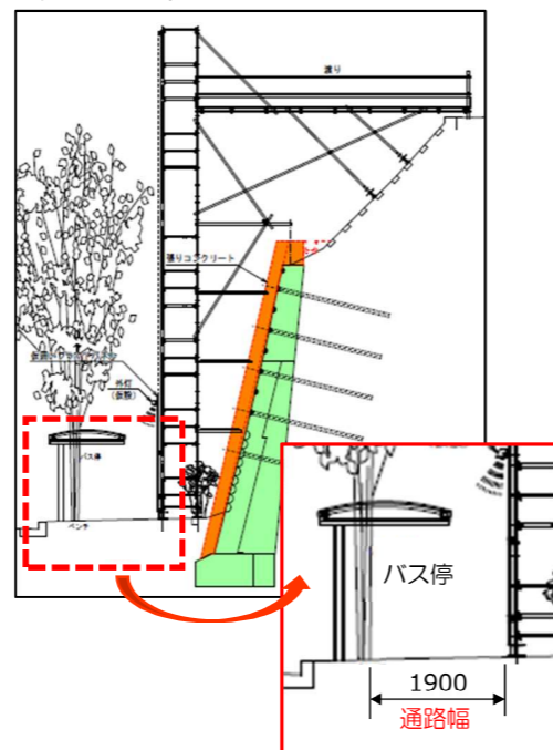
▼ 工事期間中の東側道路擁壁沿い歩道通路幅
